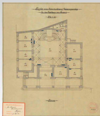
Grundriss des Hochparterres des Rathauses, erster Entwurf, Wilhelm Kürschner, 1902
