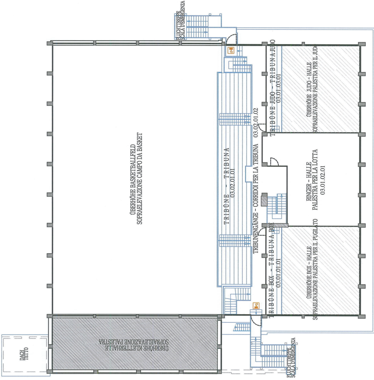
2. S T O C K SECONDO PIANO 1:200
